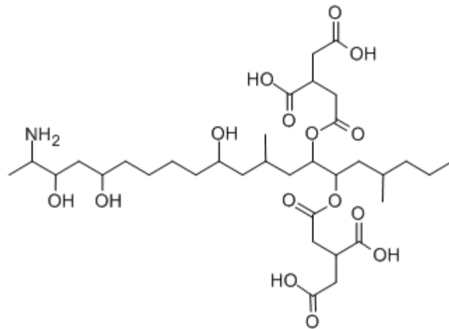
Fumonisin B1, C 34 H 59 NO 15 , Molekulargewicht 721.83 g/mol
