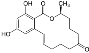
Zearalenone (ZON)
